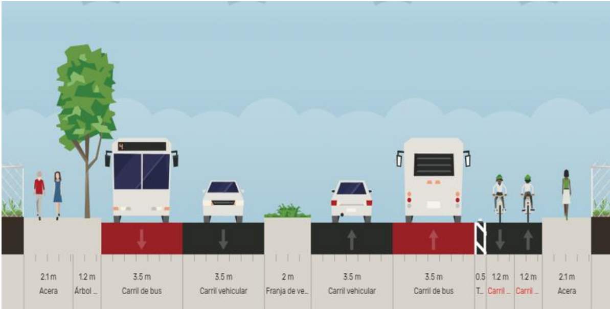
IMAGEN: PERFIL VIAL PROYECTADO
